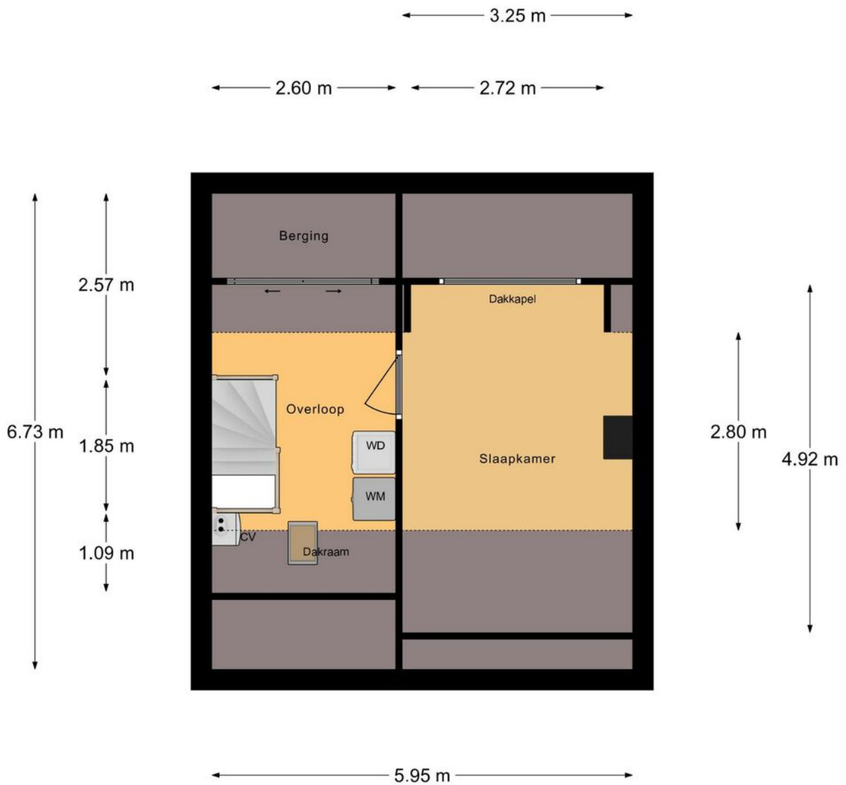
2e Verdieping
